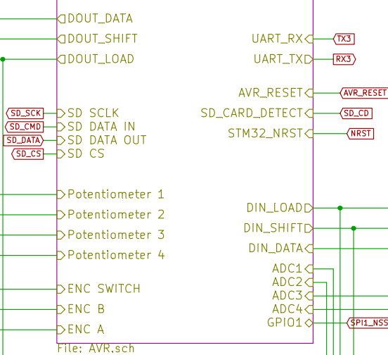
Sheet: AVR
